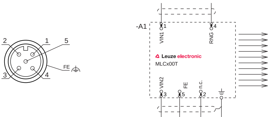
Fig. 7.2: Affectation des broches et schéma de raccordement de l'émetteur
