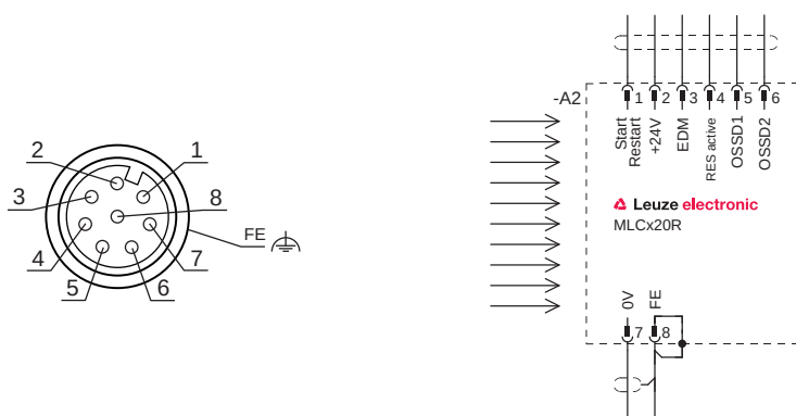
Fig. 7.4: Affectation des broches et schéma de raccordement du récepteur
