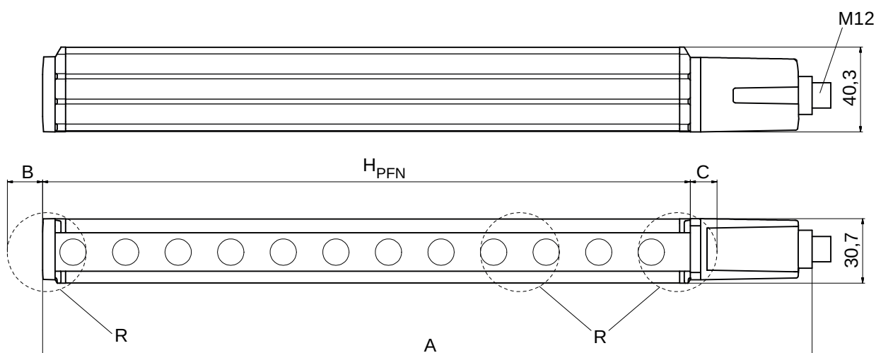
Figura 14.1: Medidas del emisor y receptor
