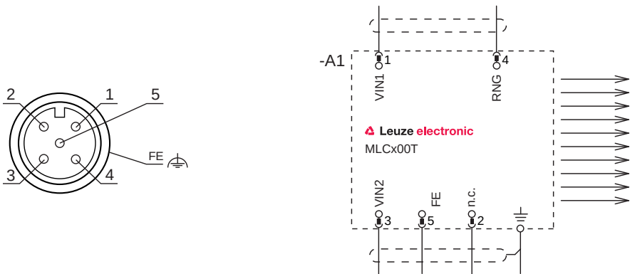
Figura 7.2: Asignación de pines y esquema de conexiones del emisor
