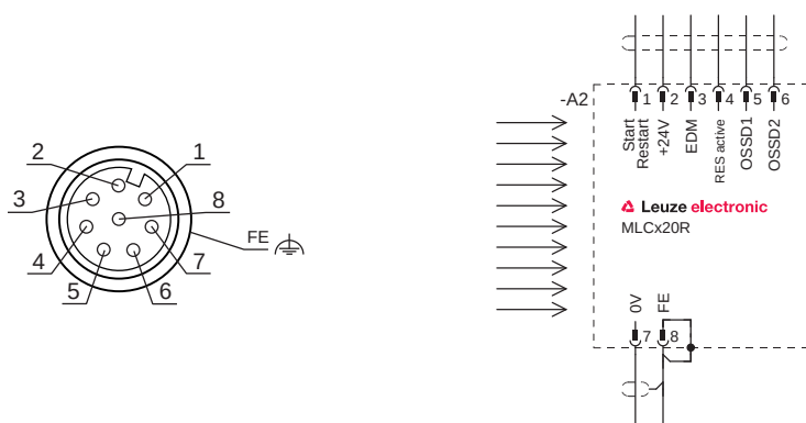
Fig. 7.3: Ocupação de pinos e diagrama de conexões do receptor
