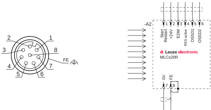
Figura 7.3: Assegnazione dei pin e schema di collegamento ricevitore
