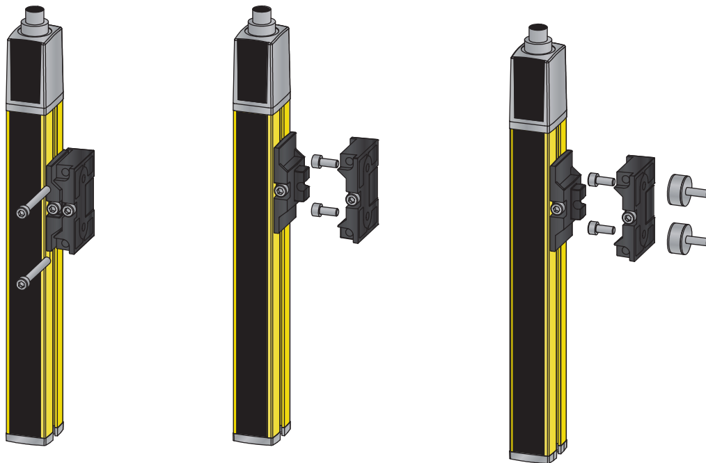
Figura 6.9: Montaje a través de soporte orientable BT-2SB10
