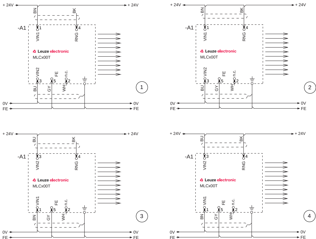
Fig. 7.2: Exemplos de conexão do transmissor
