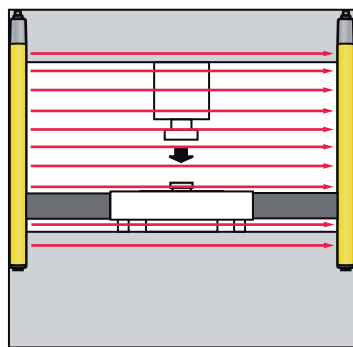
Figura 5.2: Blanking fisso: bloccaggi meccanici impediscono interventi laterali nel campo protetto
