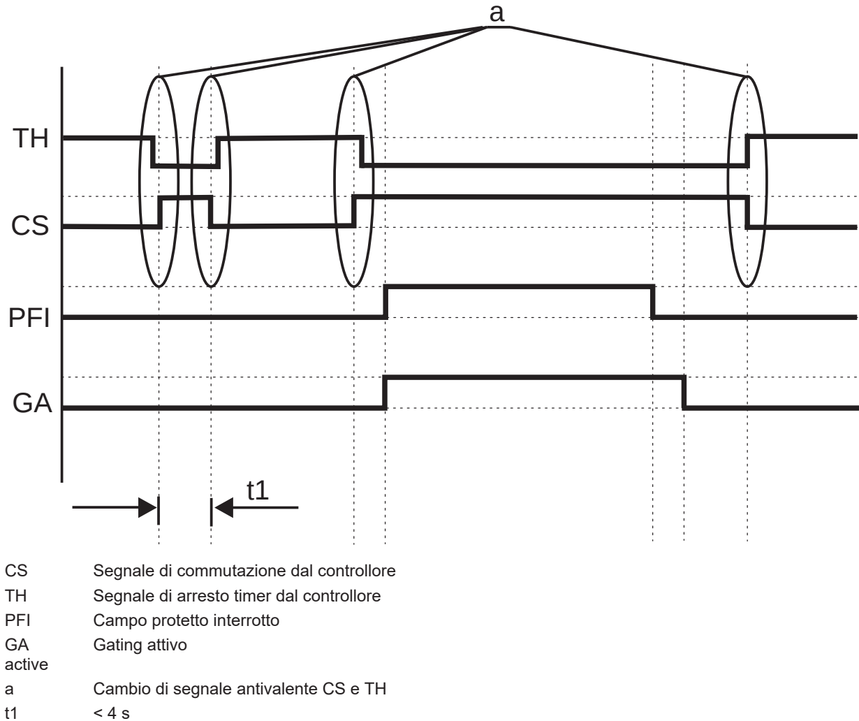
Figura 4.4: Modo operativo 1 - Arresto qualificato
