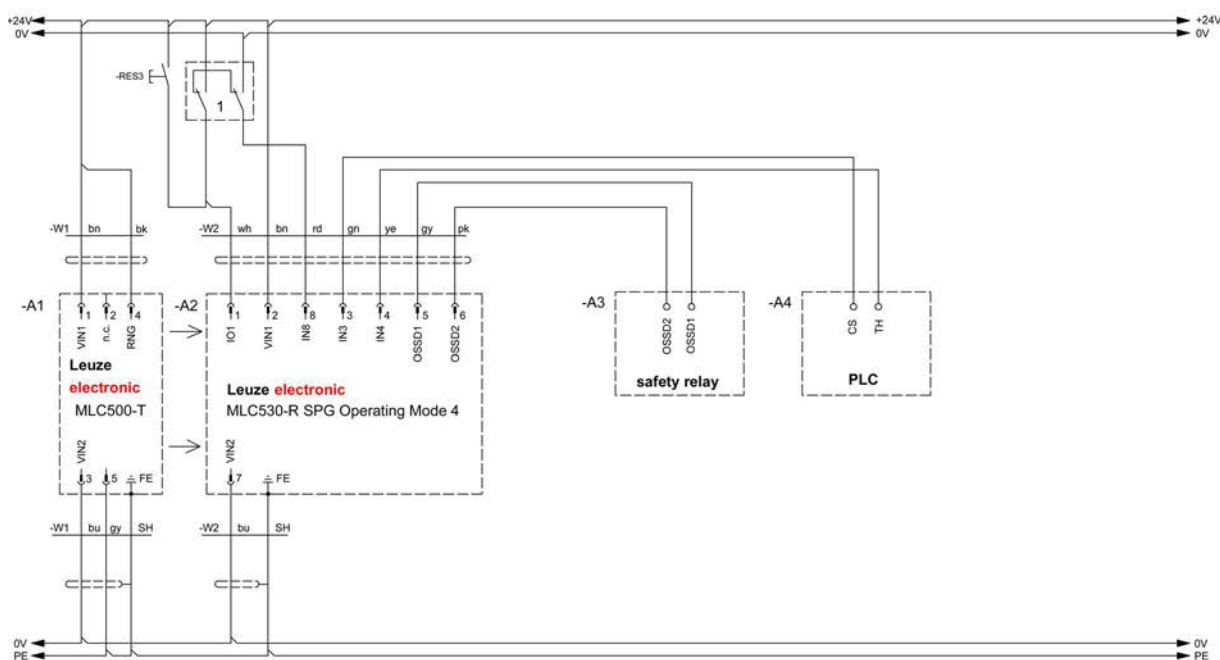
Figura 8.5: Modo operativo 4: esempio di collegamento con Smart Process Gating (SPG)
