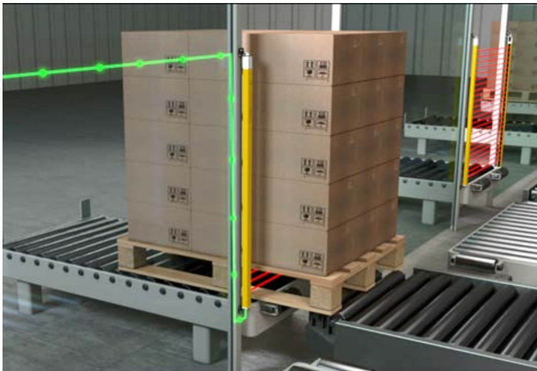
Figura 6.2: Smart Process Gating (SPG) sul percorso di trasporto
