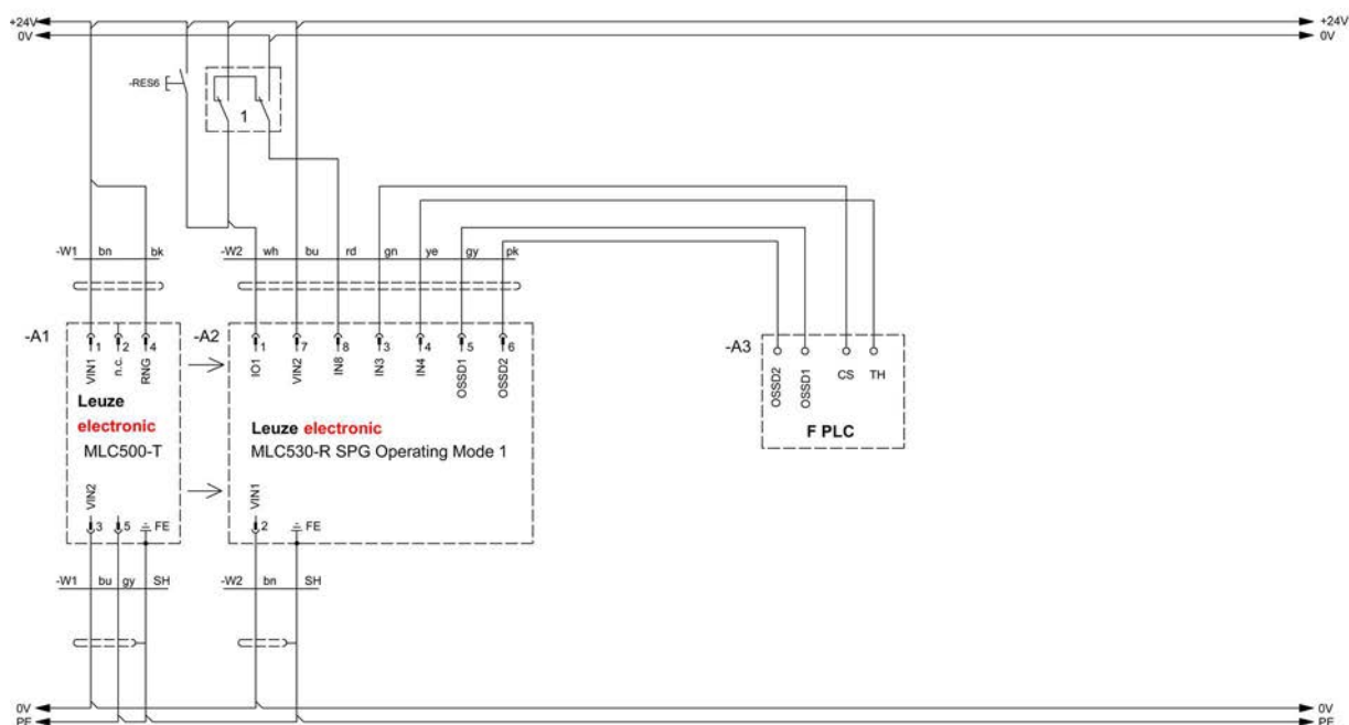
Figura 8.4: Modo operativo 1: esempio di collegamento con Smart Process Gating (SPG)
