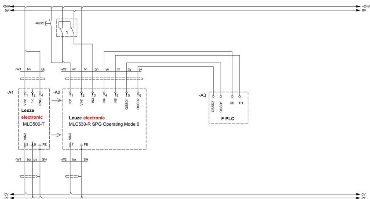
Figura 8.7: Modo operativo 6: esempio di collegamento con Smart Process Gating (SPG)
