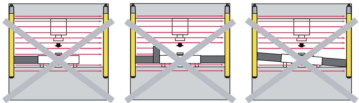
Figura 5.3: Blanking fisso: prevenzione della «formazione d'ombra»
