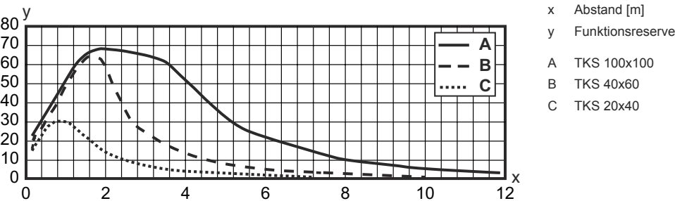
Typ. Funktionsreserve
