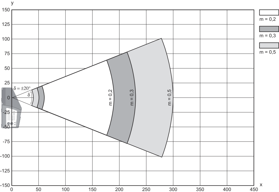
Seitliche Lesefeldkurve
