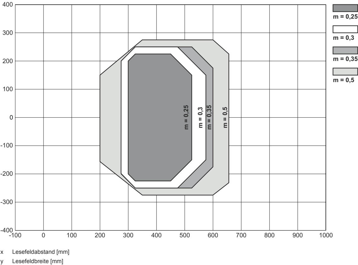
Lesefeldkurve
