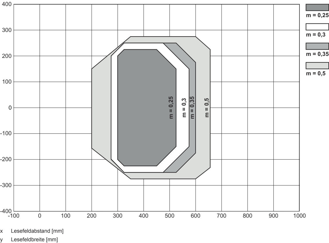
Lesefeldkurve
