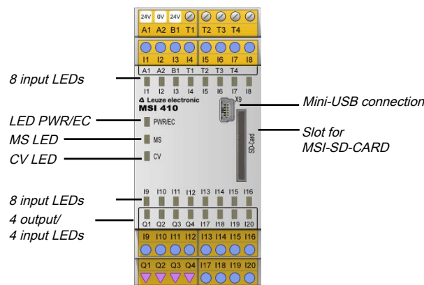
Fig. 3.3: MSI 410 display element
