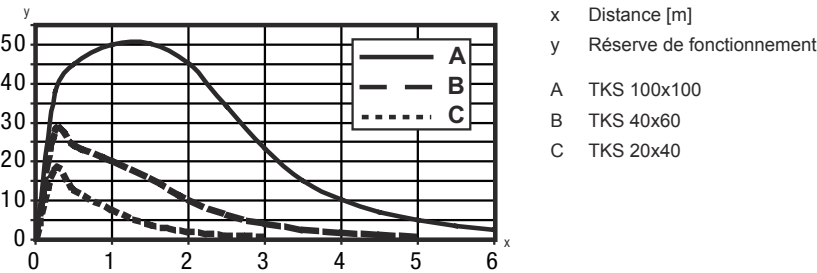
Réserve de fonctionnement typ. (variante axiale)
