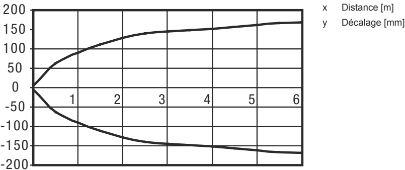
Réaction typ. (TK 100x100)
