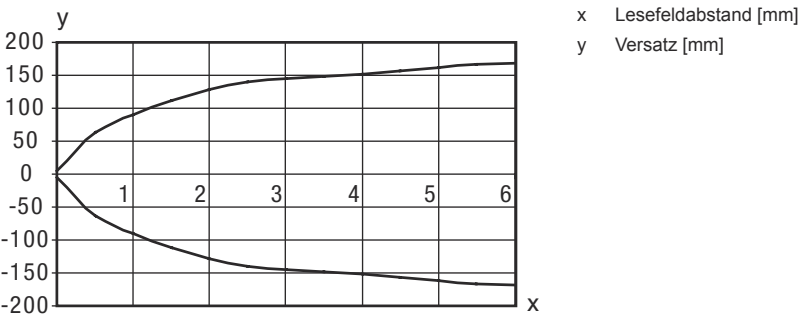
Typ. Ansprechverhalten (TKS100x100)
