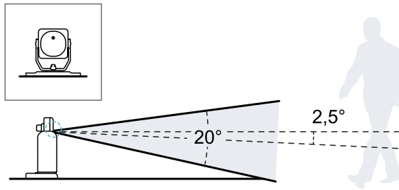
传感器倾斜度为 0^\circ 的侧视图。
