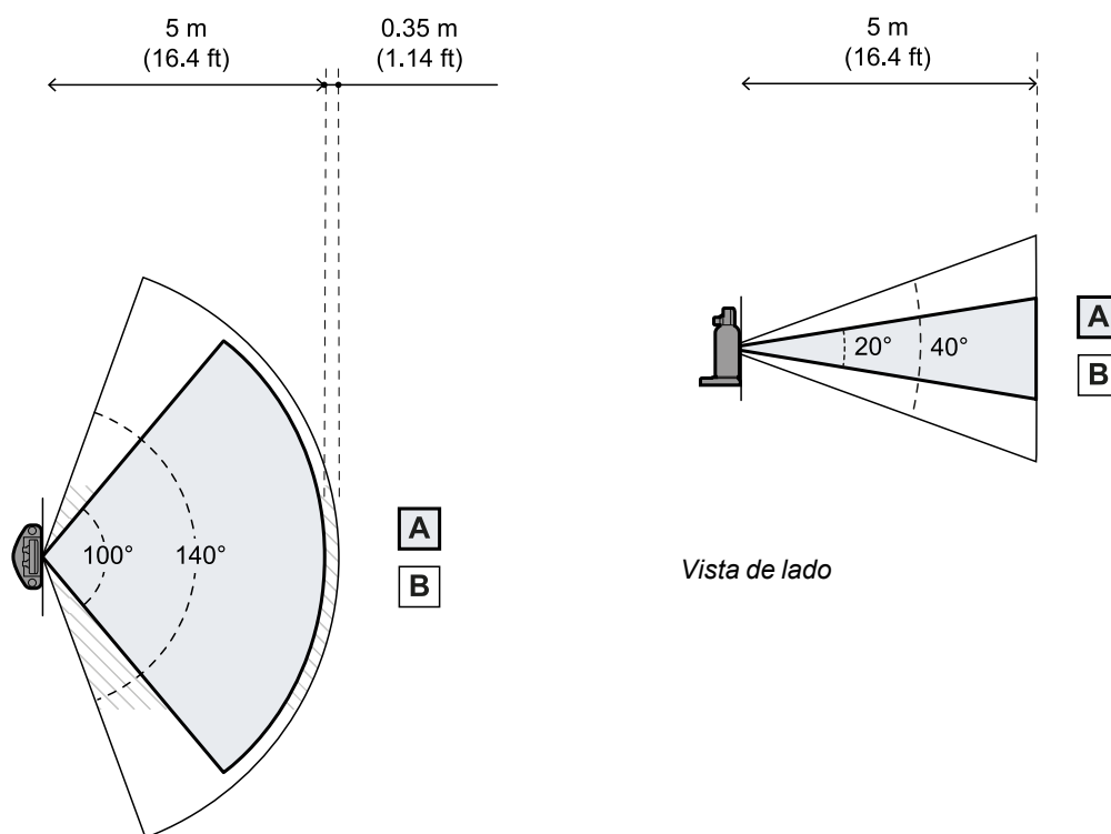
Vista de cima
