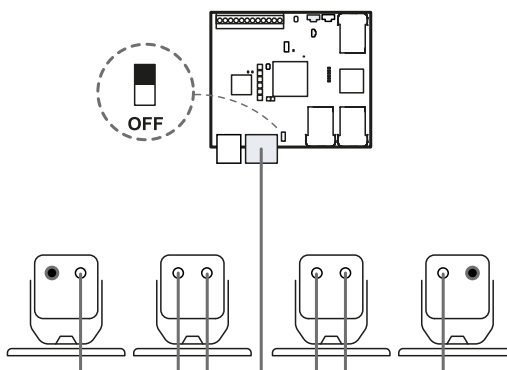
Cadeia com unidade de controle no interior dela e dois sensores com terminação bus
