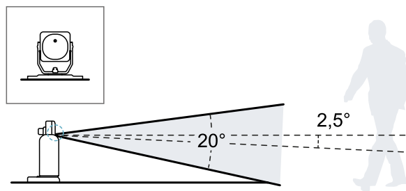
Vista lateral com inclinação do sensor a 0°.
