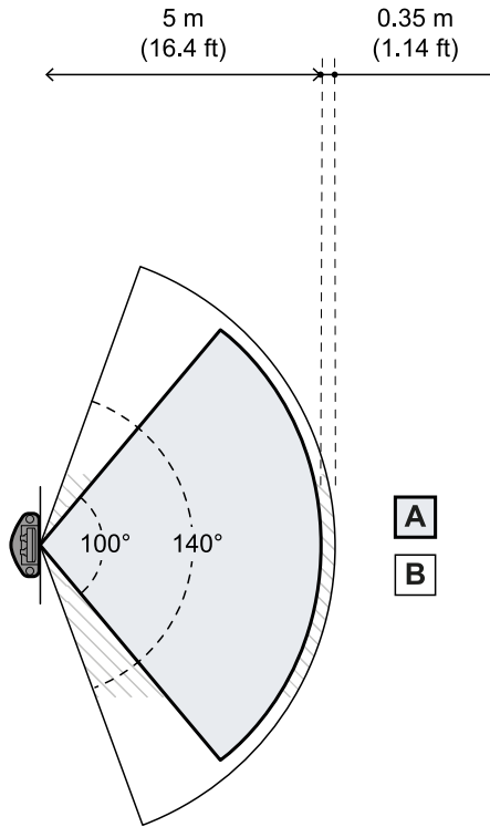
상면도
