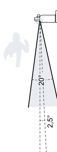
Vista desde arriba con inclinación del sensor a 0^\circ .
