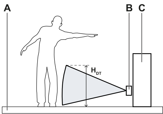
Ejemplo de H_{DT} \leq 1000 mm (acercamiento paralelo)
