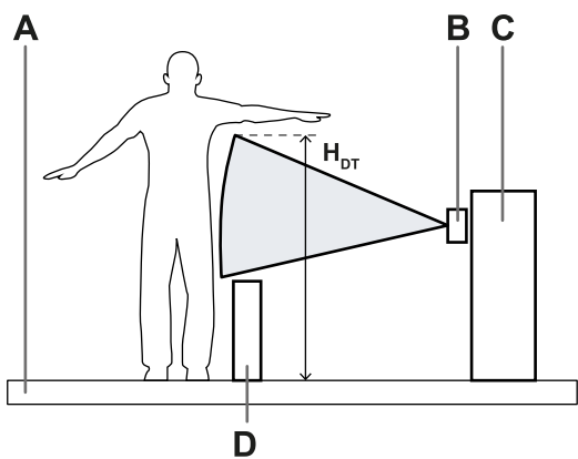
Ejemplo de H_{DT} \geq 1400 mm (aproximación paralela)
