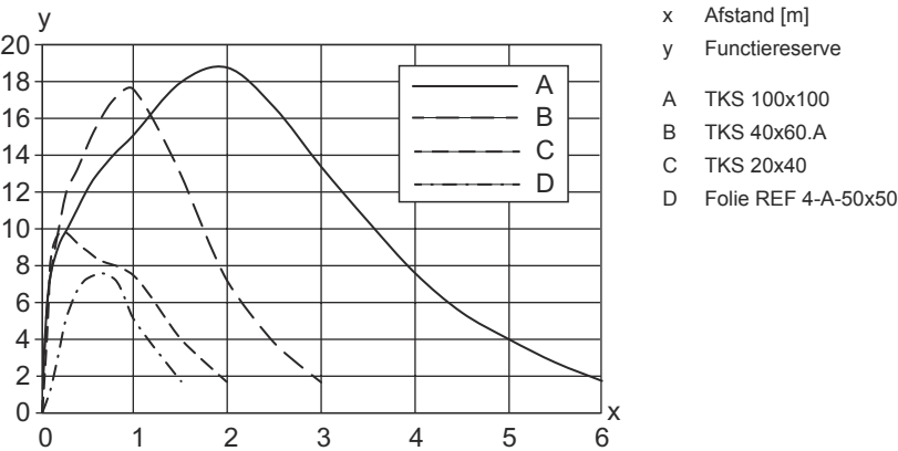
Typische functiereserve
