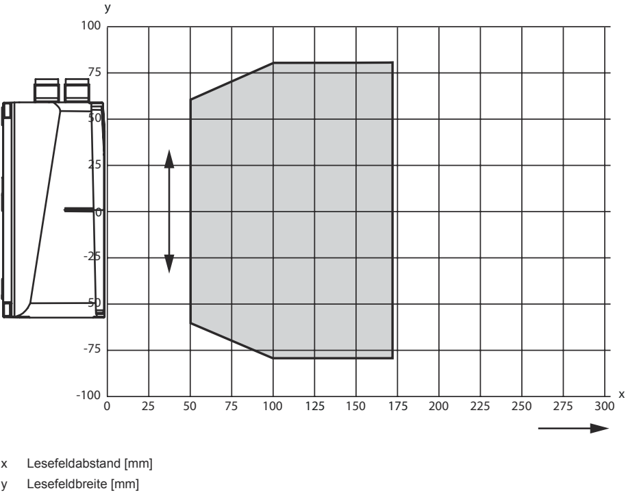
Lesefeldkurve
