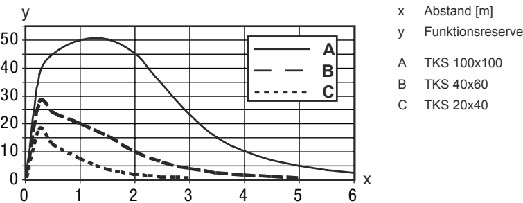
Typ. Funktionsreserve
