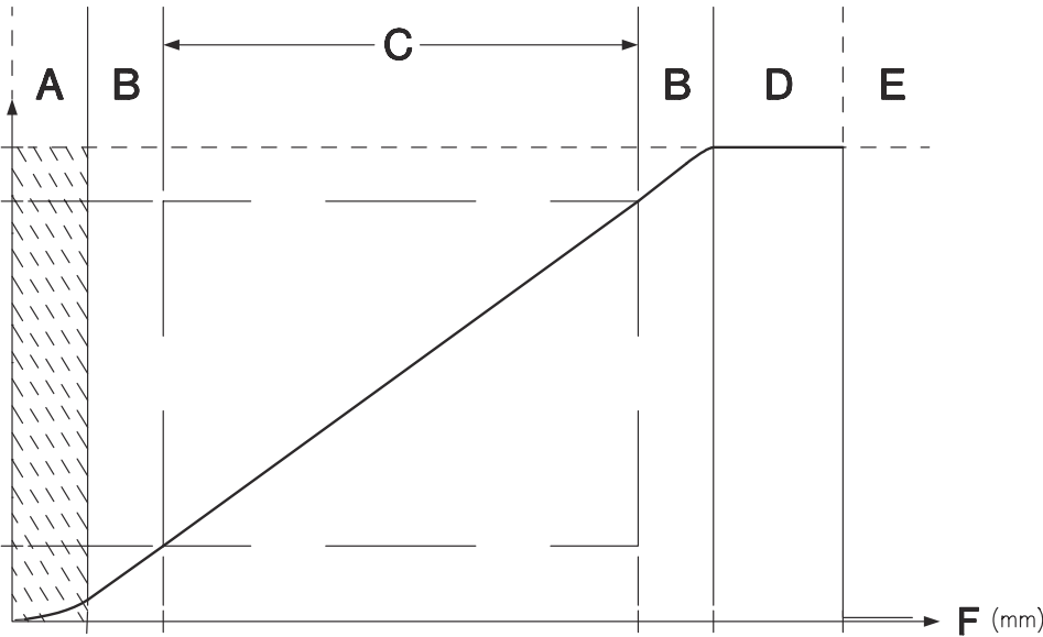
Caractéristique de sortie de la sortie analogique
