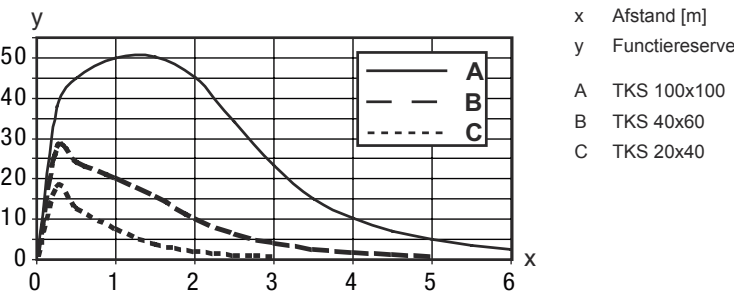
Typische functiereserve
