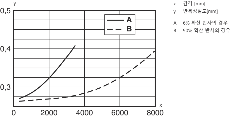
반복정밀도 유형 측정 모드 "최고 정밀"
