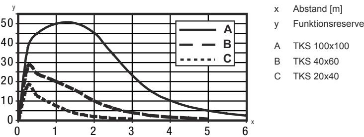
Typ. Funktionsreserve
