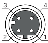
图 7.3: 以太网接口引线布局
