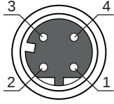
Resim 7.3: Ethernet arayüzü bağlantı düzeni
