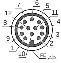
Resim 7.2: M12 konektör, 12 kutuplu, A kodlu bağlantı yerleşimi
