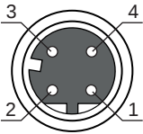
Fig. 7.3: Pinagem de interface Ethernet
