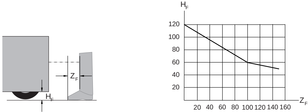
그림 6.14: 바닥의 빈 공간 H_F 가 부족할 때 여유한계 H_F 를 결정하기 위한 도표
