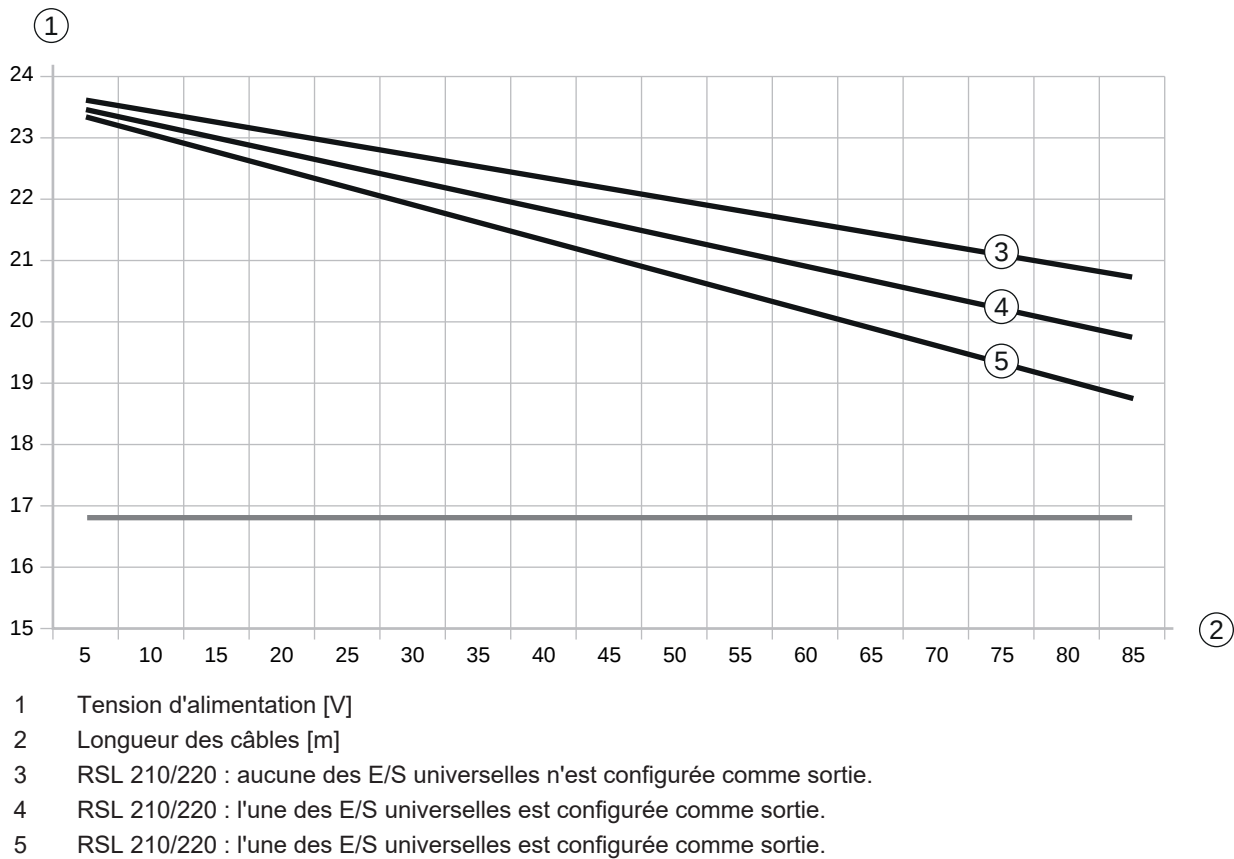
Fig. 7.1: Schéma d'estimation de la chute de tension sur la ligne d'alimentation (section de ligne = 0,25 mm² ( câble à 8 broches))
