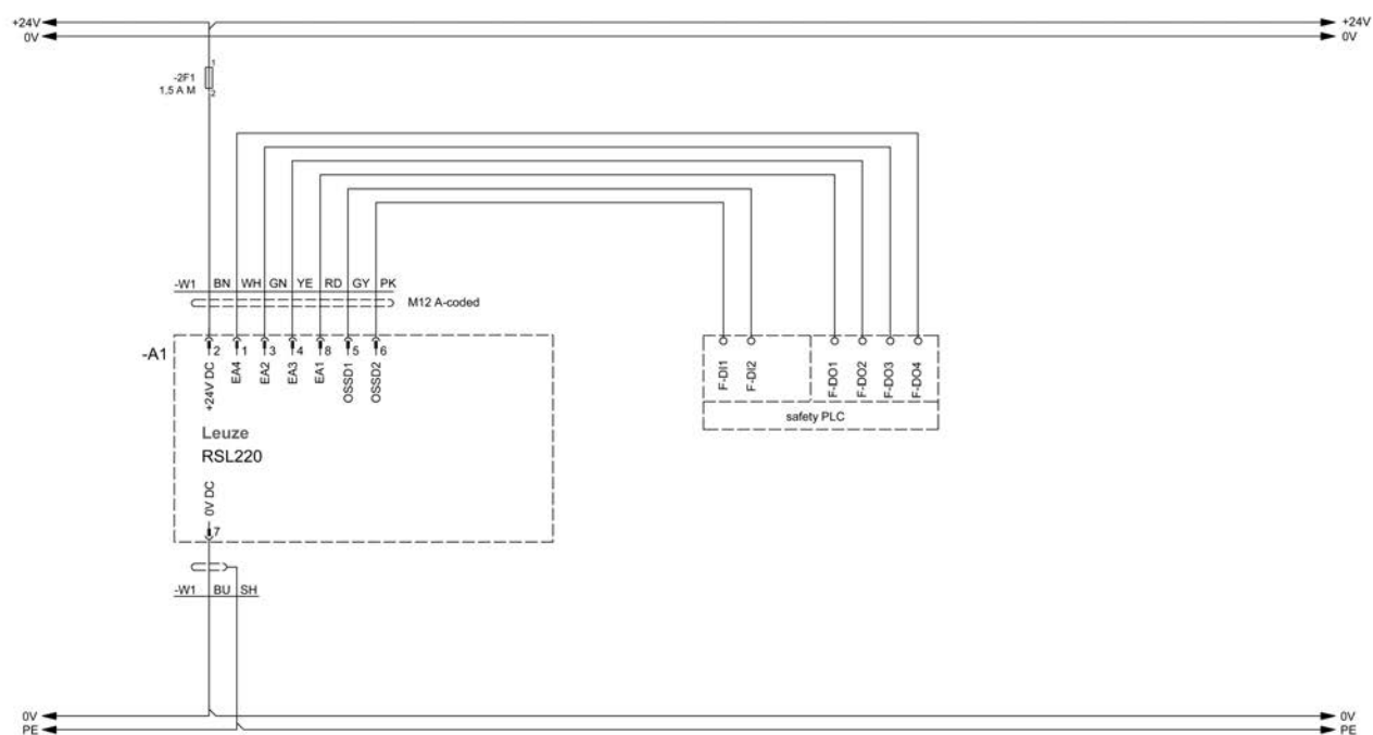
Fig. 7.3: RSL 220 avec contrôleur de sécurité
