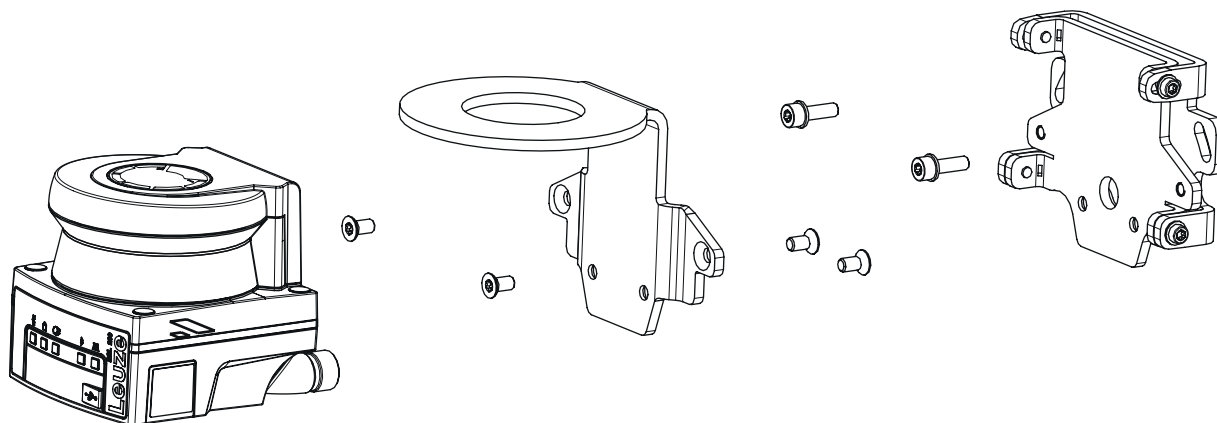
Fig. 6.17: Montage avec support mural et support de protection
