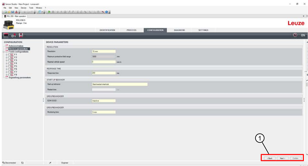
Fig. 8.5: Configuration de sécurité avec l'assistant de configuration
