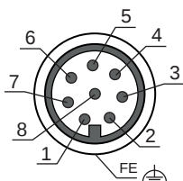
Fig. 7.2: Affectation des raccordements du connecteur M12, 8 pôles
