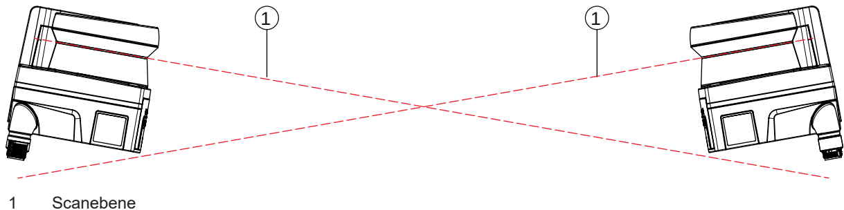
Bild 6.9: Montage gegenüberliegend, ohne Höhenversatz, gekreuzte Ausrichtung
