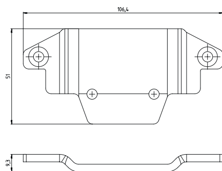
Bild 14.2: Montagesystem BTU 500M
