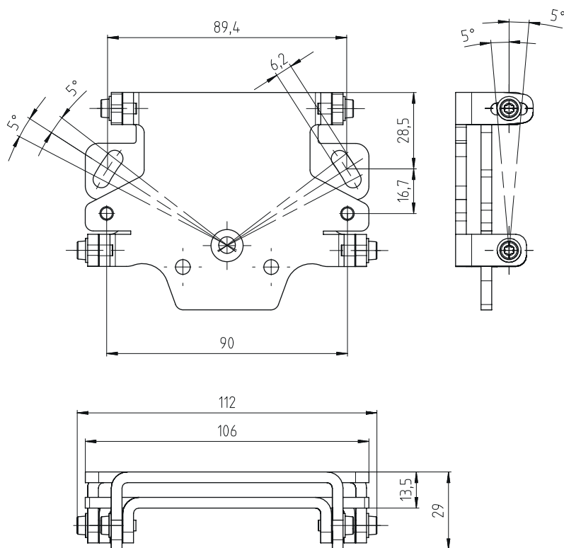
Bild 14.2: Montagesystem BTU 500M
