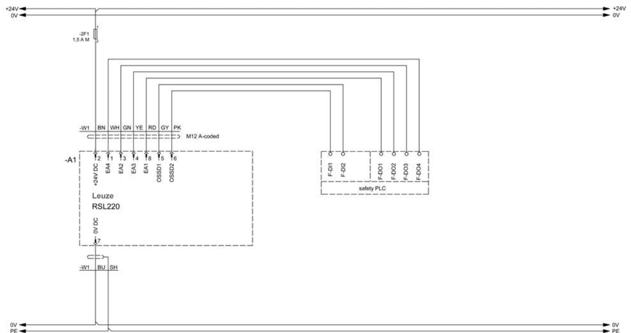
Bild 7.3: RSL 220 mit Sicherheits-Steuerung
