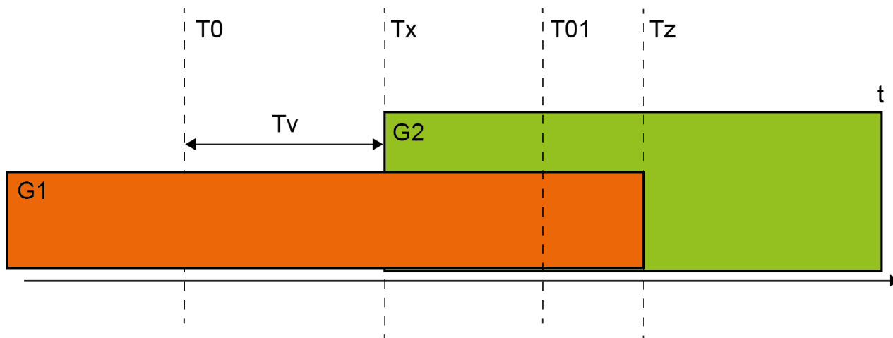
Bild 4.7: Schutzfeldumschaltung bei 2 Gefahrenstellen
