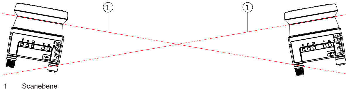
Bild 6.8: Montage nebeneinander, ohne Höhenversatz, gekreuzte Ausrichtung
