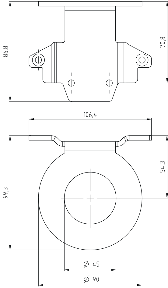
Resim 14.4: Koruma demiri BTP 500M
