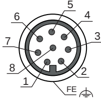
Resim 7.2: M12 konnektör, 8 kutuplu bağlantı yerleşimi
