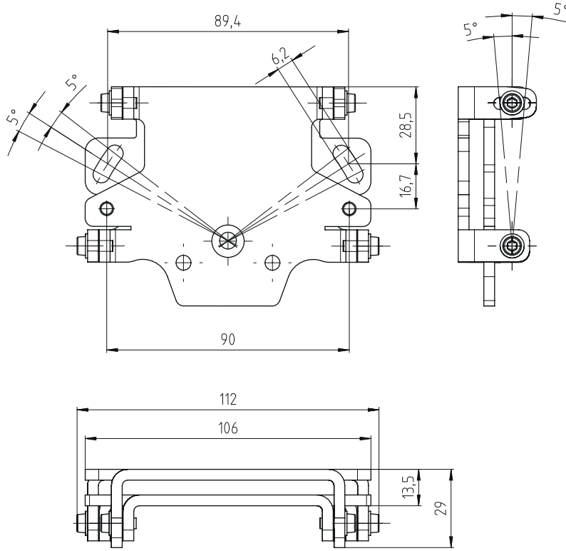
Resim 14.2: BTU 500M montaj sistemi
