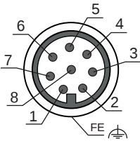
Fig. 7.2: Pinagem Conector M12, de 8 polos
