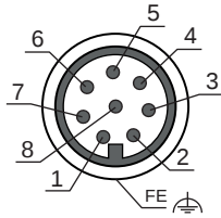
그림 7.2: M12 커넥터 연결부 할당, 8핀
