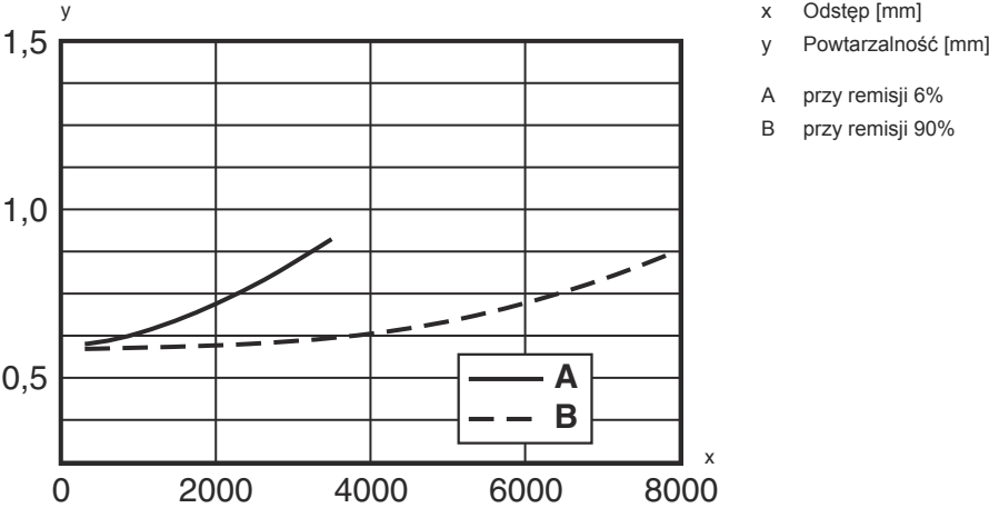
Typ. powtarzalność w trybie pomiarowym "wysoka precyzja"
