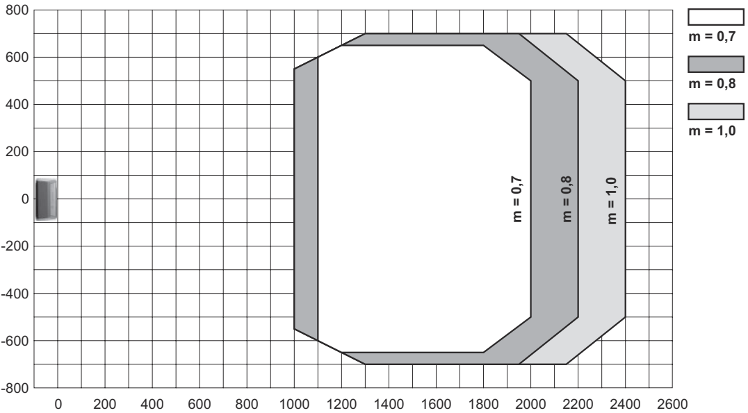
Krzywa pola odczytu
