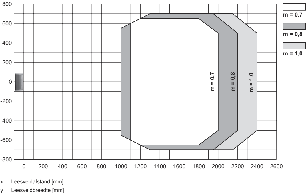
Leesveldcurve
