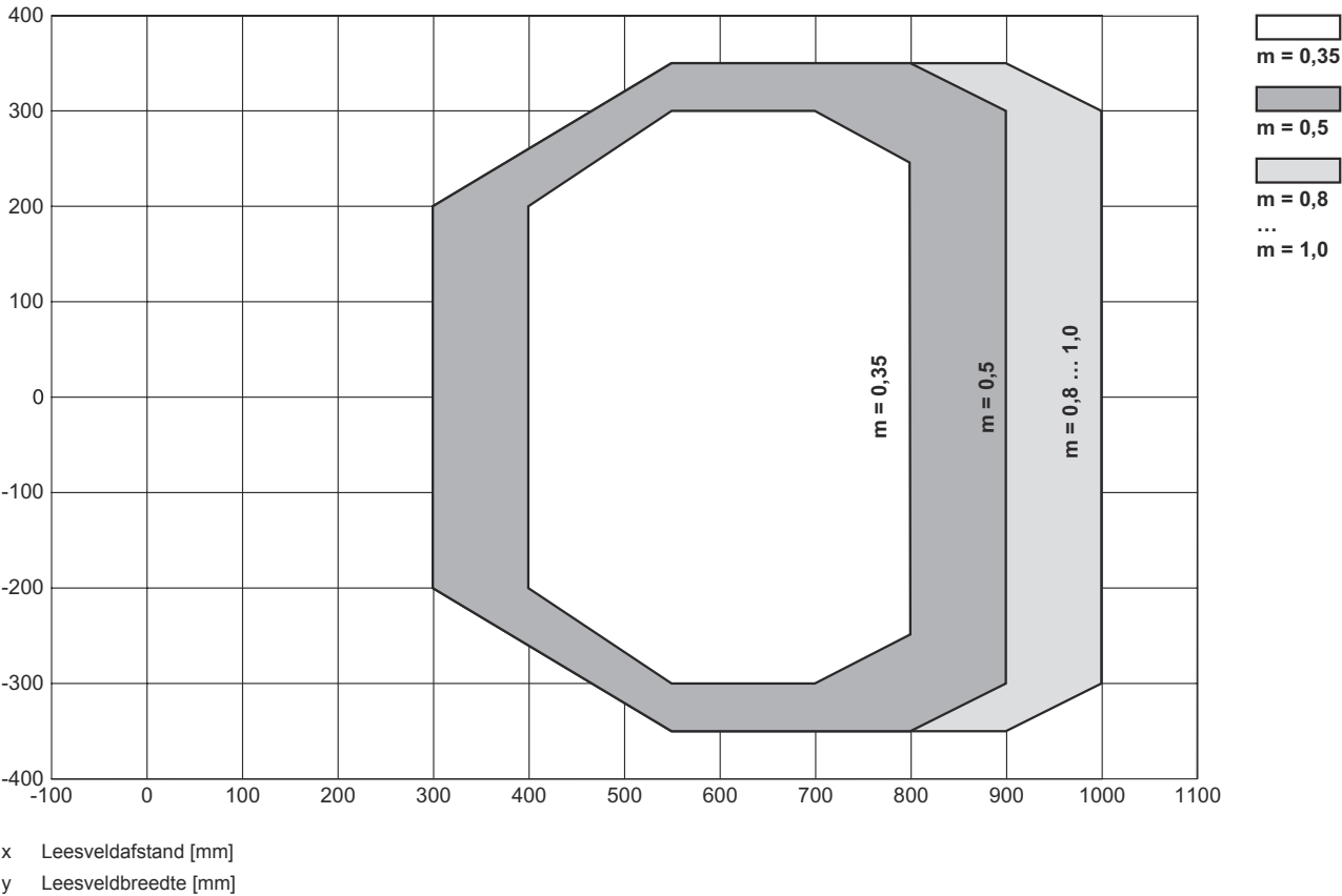
Leesveldcurve
