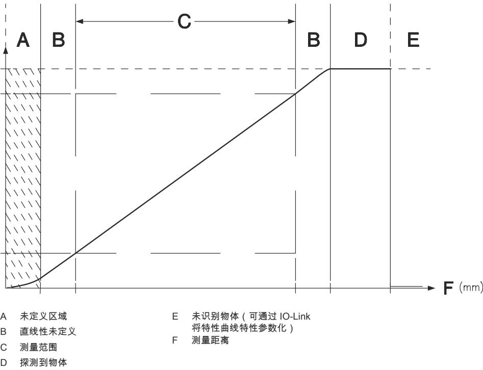
模拟输出端输出特性曲线
