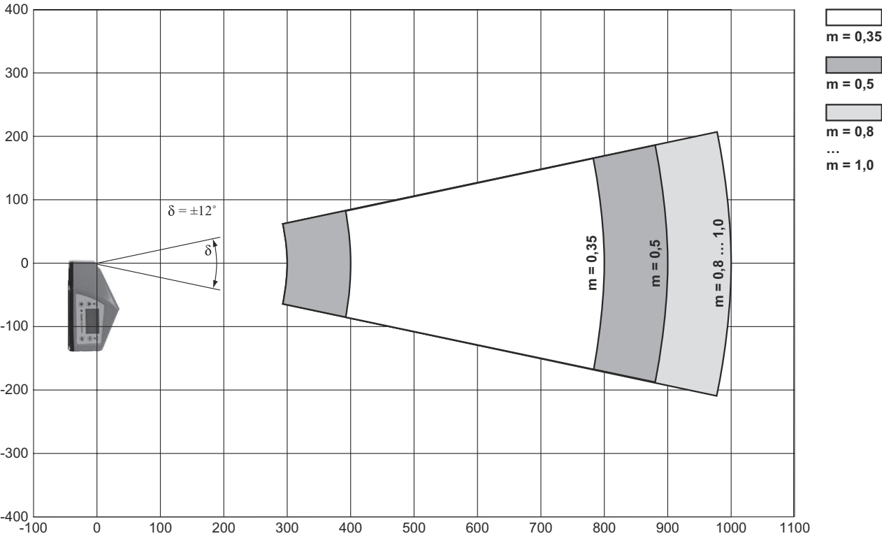
侧面条码阅读曲线
