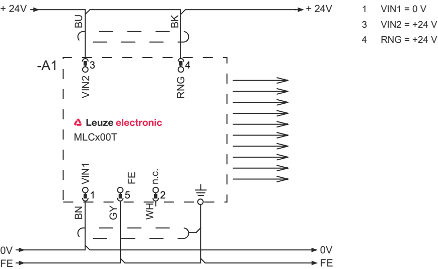
传输通道 C2，接收器上的 OSSD 已激活
