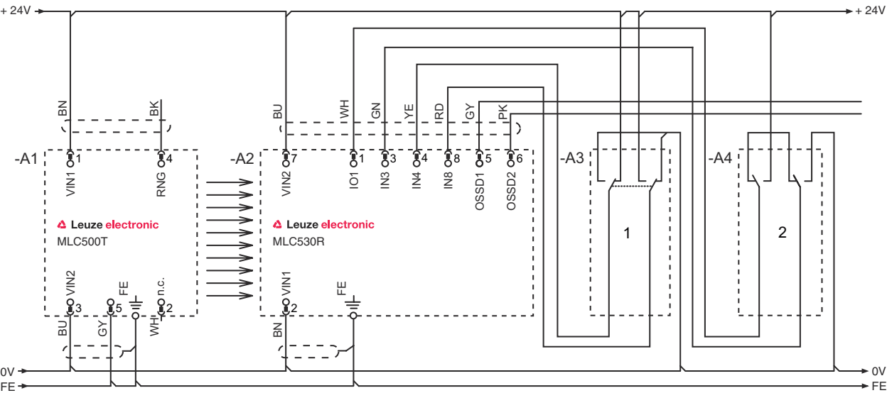
Conmutador de llave para conmutar entre los grupos de funciones FG1 y FG2 Interruptor con llave para el aprendizaje de zonas de blanking
