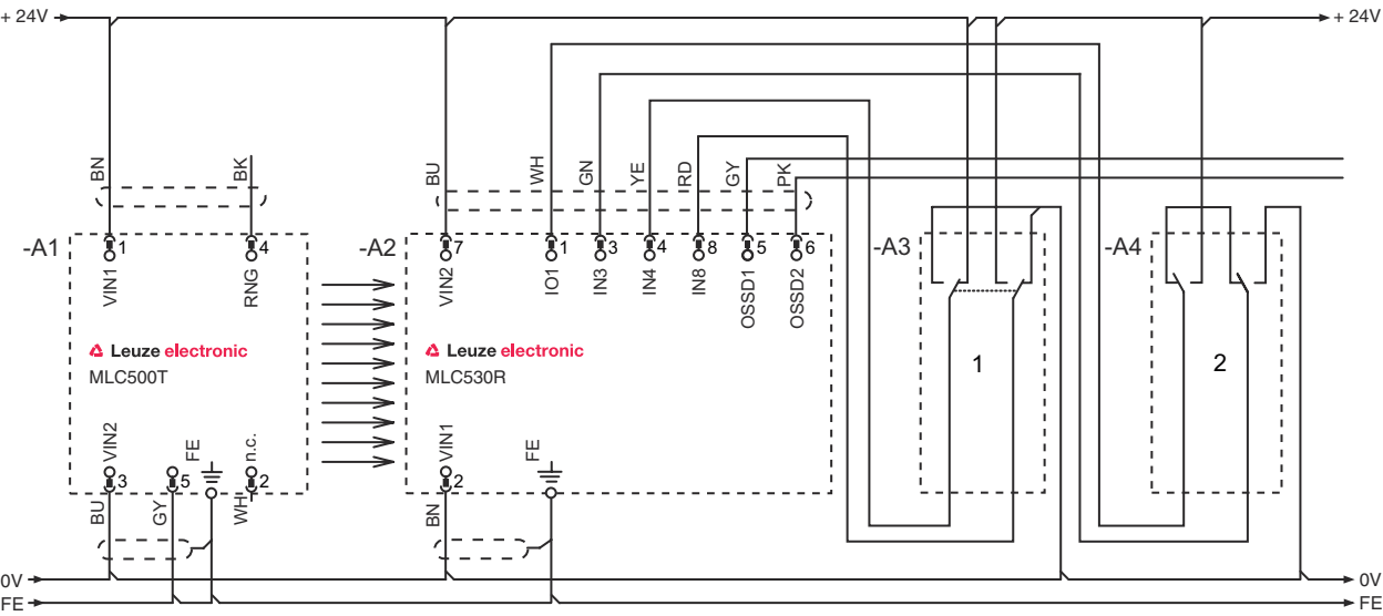
Interruptor de chave inversor para alternar entre os grupos funcionais FG1 e FG2 Interruptor de chave para programação de faixas de blanking
