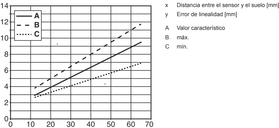
Curva característica del valor típico: error de linealidad
