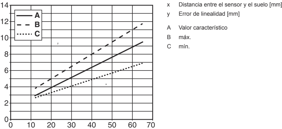
Curva característica del sensor en una pista
