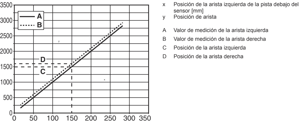
Curva característica del sensor en una pista
