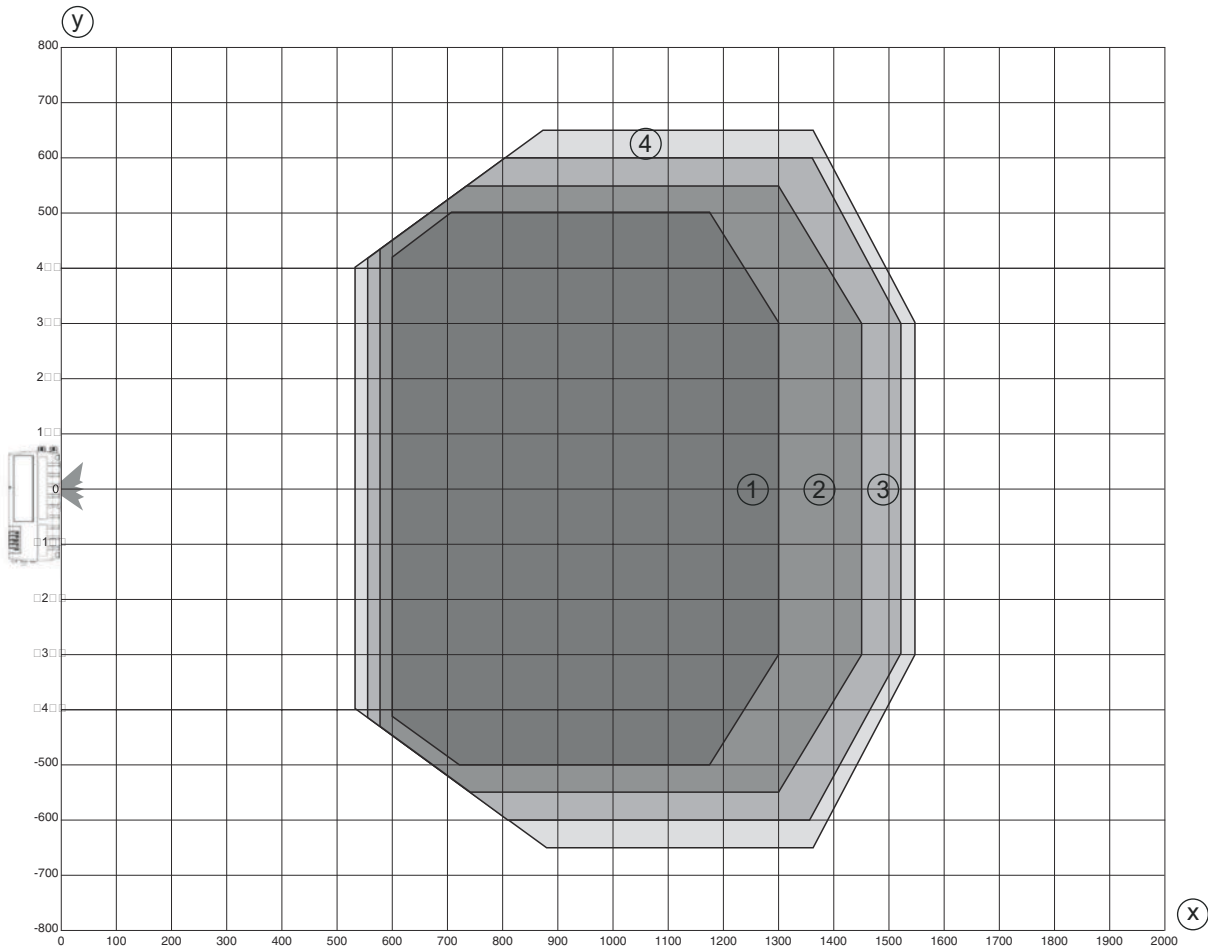
Curva del campo de lectura High Density
