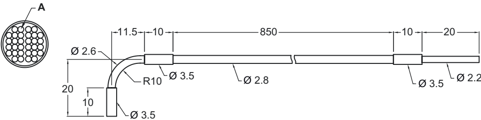
A Ø 0,265 mm núcleo de fibra de vidrio x 32 uds.
