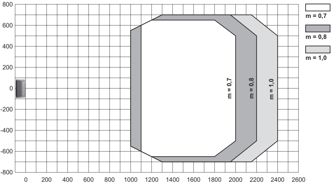
Curva del campo di lettura
