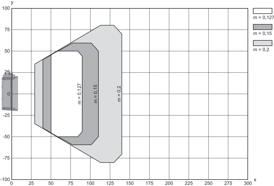
Lesefeldkurve
