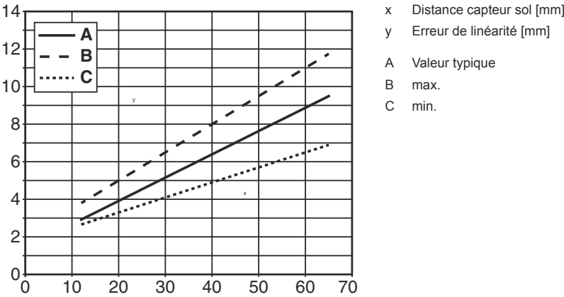
Courbe caractéristique de valeur typique : erreur de linéarité
